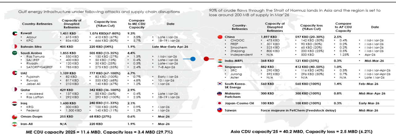
그림 1. 중동/아시아 정제설비 생산차질 현황
